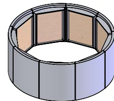
Keramický prstec. Volitelně je možné přidat další či jen vyplnit kachle šamotem pro zvýšení akumulace
